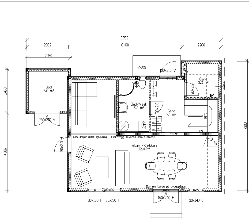
Plan 1. etasje. BYA=64,8m 2 / BRA=57,2m 2
