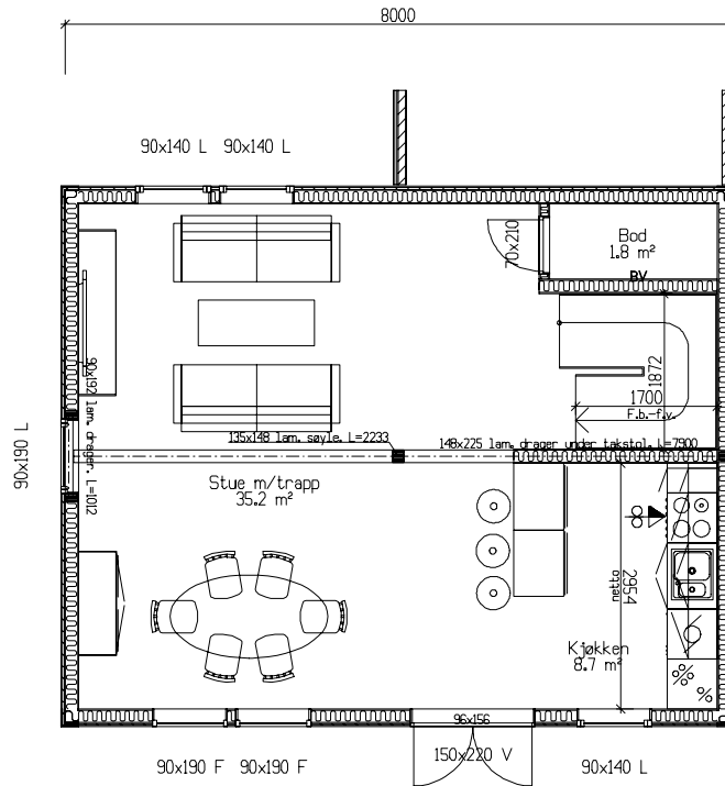
Plan 2. etasje. Bra=46,7m 2
