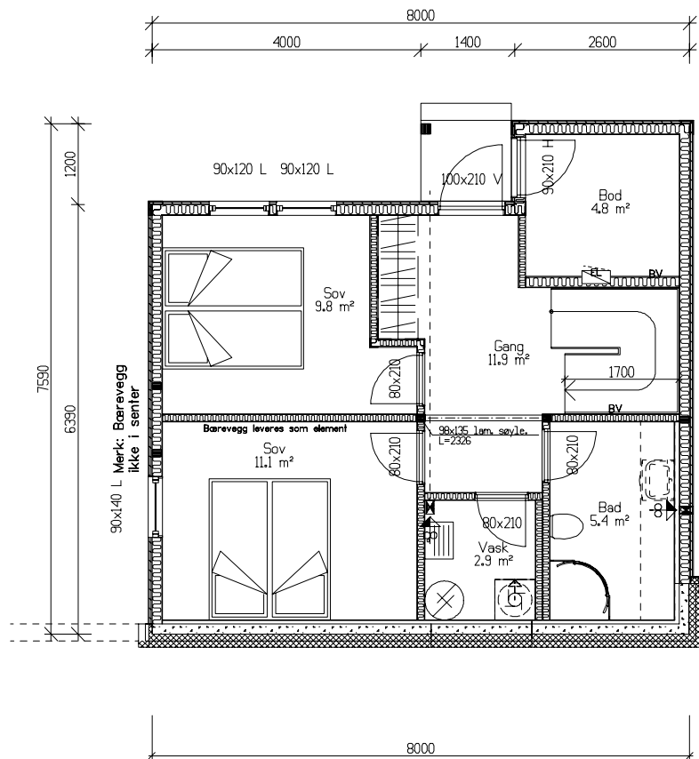
Plan 1. etasje Brutto=56,2m 2 / Bra=49,4m 2
