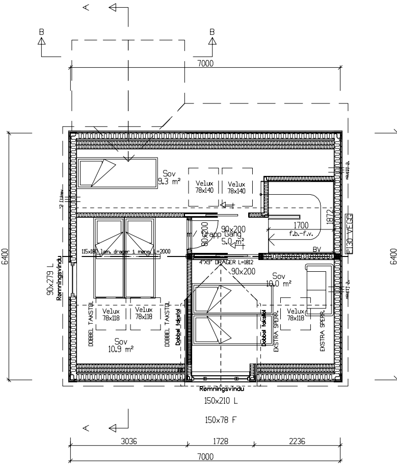
Loftsplan Bra=26,6m 2
