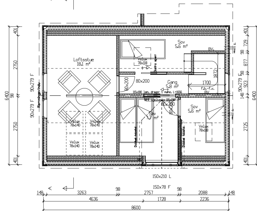
Loftsplan Bra=32,5m²
