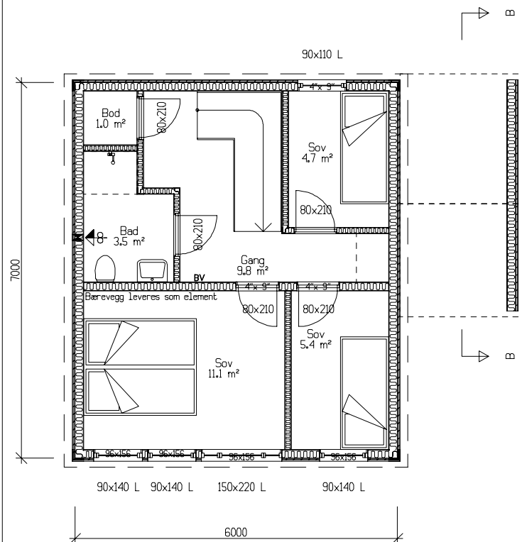
Plan 2. etasje. Bra=37,9m 2
