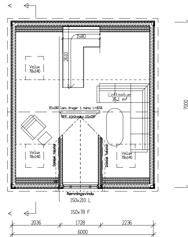
Loftsplan Bra=23,9m 2
