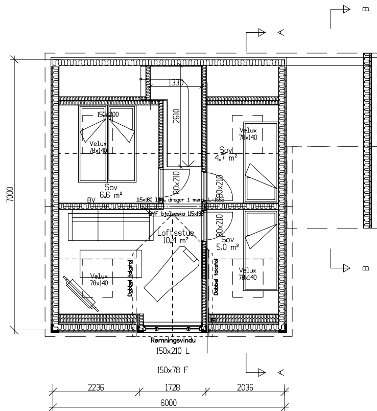
Loftsplan Bra=23,9m 2
