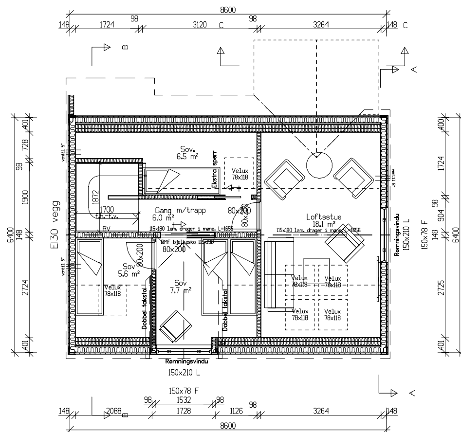
Loftsplan Bra=32,5m 2
